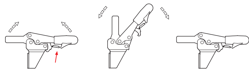
Funktionsprinzip
