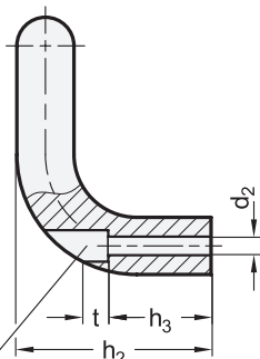
Bohrung für Zylinderschraube ISO 4762
