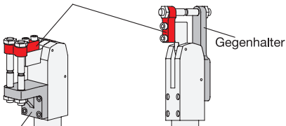
Spannbackenhalter
