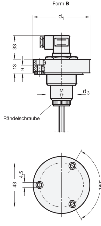
Form A mit Gewinde B mit Befestigungsflansch
