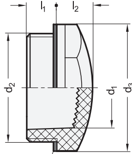
Dichtung aufliegend
