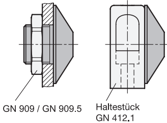
Montagebeispiele
