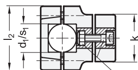
Zylinderschraube / Sechskantmutter
