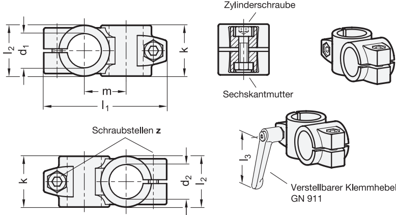
4 Kennziffer 2 mit 2 Edelstahl-Zylinderschrauben DIN 912
